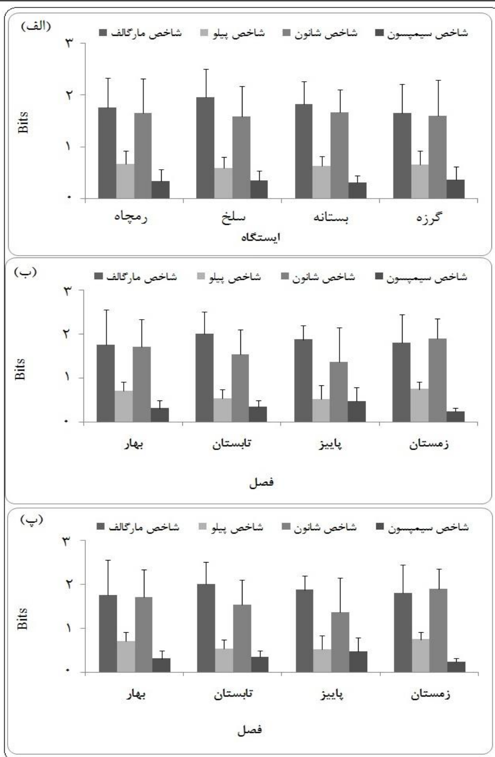
شکل ۳: تغییرات میانگین (Mean±SE) شاخص های زیستی محاسبه شده به تفکیک ایستگاه (الف) و فصل در دو منطقه قشم (ب) و بندر لنگه (پ)
