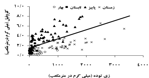
شکل ۲: ارتباط غلظت کلروفیل-آ و زی توده فیتوپلانکتون (الف) و ارتباط محتویات کلروفیل-آ سلول فیتوپلانکتون با سایز سلول (ب) در دریای خزر - منطقه گهرباران، سال ۱۳۹۲
