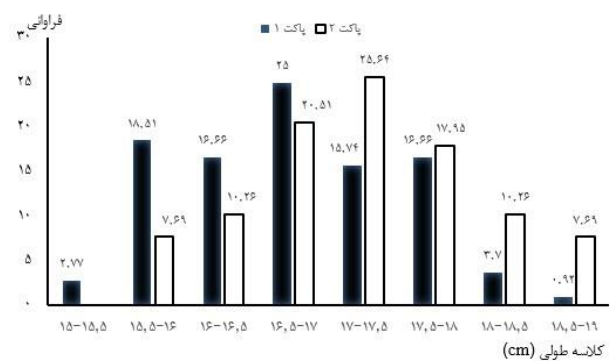
شکل ۳. فراوانی طولی ساردین روغنی ( S. longiceps ) در پاکت‌های شماره ۱ و ۲
