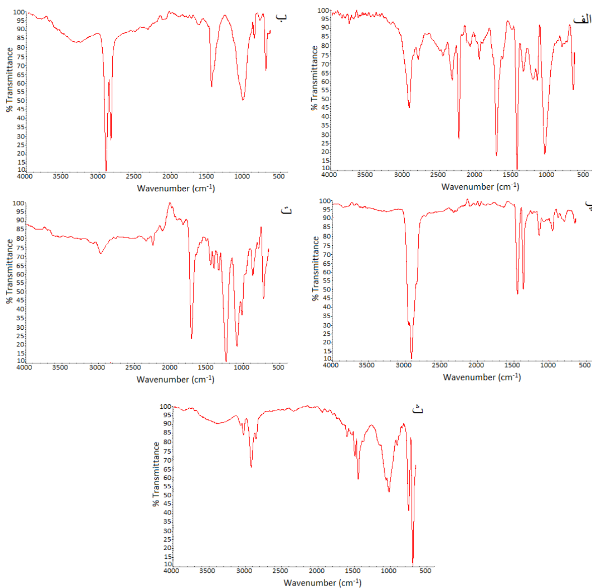
شکل ۴: پلیمرهای یافت شده در رسوبات تالاب انزلی. الف: پلی‌اکریلونیتریل، ب: پلی‌اتیلن، ج: پلی‌پروپیلن، د: پلی‌استر، ه: پلی‌استایرن Figure 4: Polymers found in the sediments of Anzali wetland. a: Polyacrylonitrile, b: Polyethylene, c: Polypropylene, d: Polyester and e: Polystyrene
