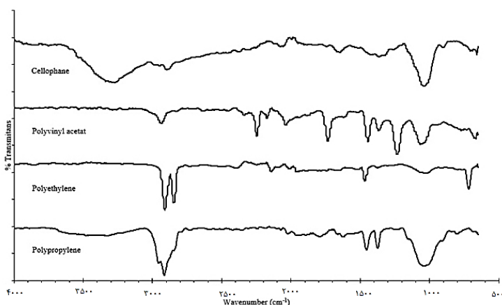
شکل ۶: طیف ATR-FTIR میکروپلاستیک‌های یافت شده در رسوبات Figure 6: ATR-FTIR spectrum of microplastics found in sediments
