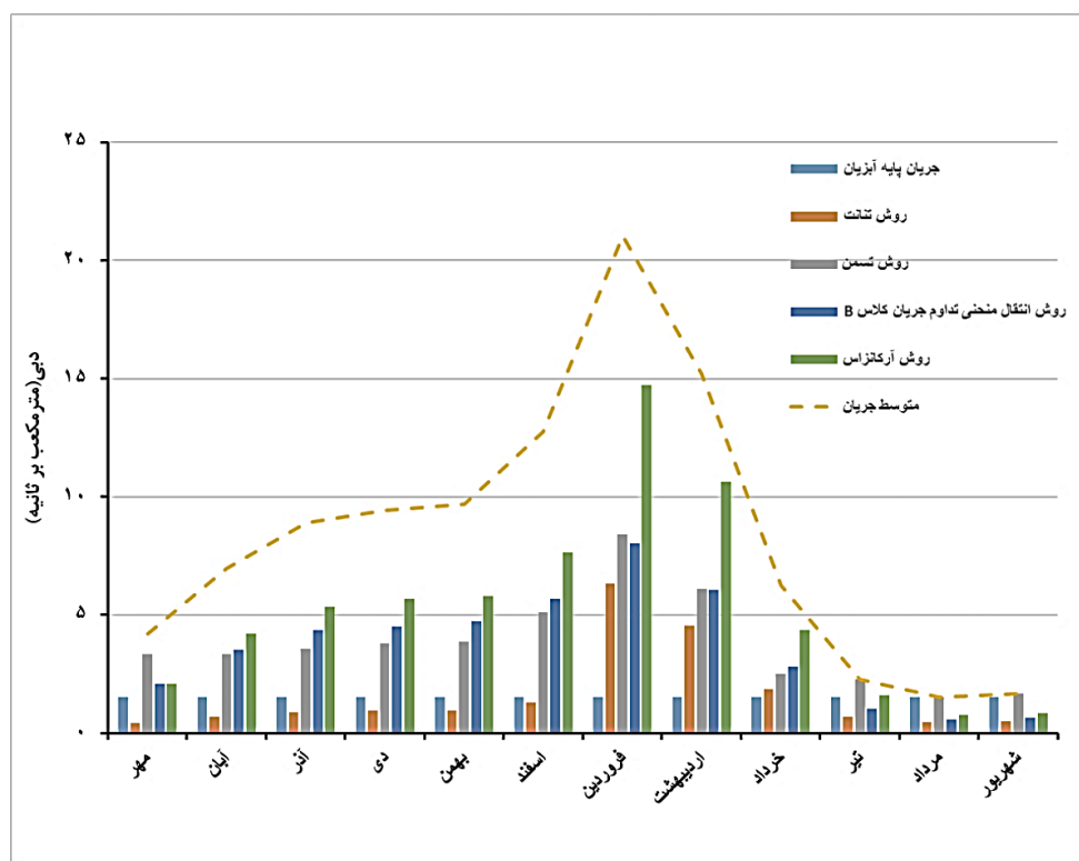
شکل ۴: توزیع ماهانه جریان زیست‌محیطی رودخانه دره‌رود - مشیران به روش‌های مختلف (مترمکعب بر ثانیه)
